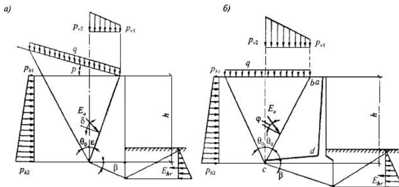
Рисунок 1 - Расчетные схемы подпорных стен
