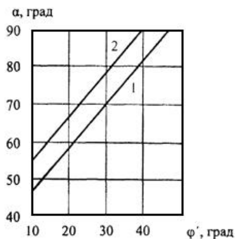
Рисунок 7 - Графики для определения угла наклона стенок бункеров для связных материалов
